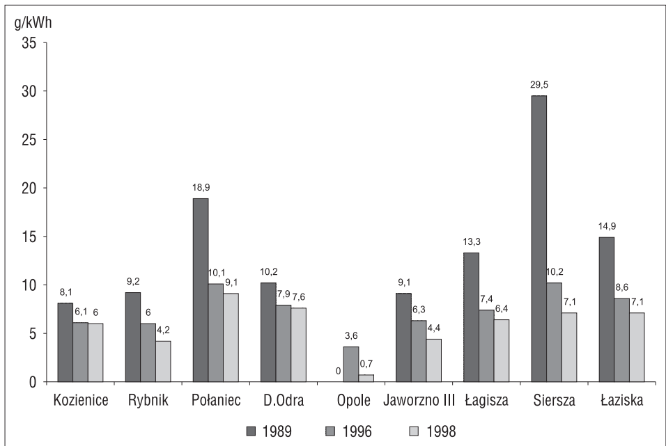
Fig. 3. Unit SO 2 Emissions in Hard-Coal Fired Plants Larger Than 700 MW in 1989, 1996 and 1998. Ryc. 3. Jednostkowa emisja SO 2 w elektrowniach na węgiel kamienny o mocy powyżej 700 MW w latach 1989, 1996, 1998
